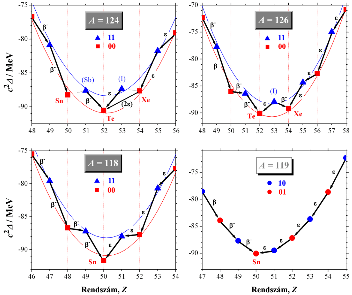
43. ábra: A 40. ábrán sárga vonallal összekötött izobár nuklidok tömegparabolái a legnagyobb stabilitás (minimum) közelében. Amint látjuk, szembejövő a különbség az egyetlen páratlan- A grafikon (jobb alsó panel) és a többi ábra közt, amelyek mind páros- A nuklidokat mutatnak. Bővebb magyarázat a szövegben. ( Jelmagyarázat: 0 = páros; 1 = páratlan; 00, 01, 10, 11 = Z & N párossága ebben a sorrendben.)
