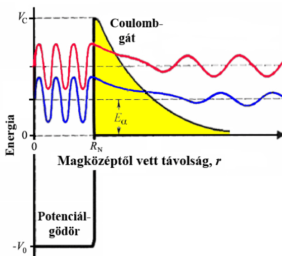
18. ábra: Egy \alpha -részecske áthatolása a mag Coulomb-gátján alagúthatás segítségével (kék hullám). Ha a részecske kinetikus energiája nagyobb lenne, akkor a hullámfüggvénye (piros hullám) kevésbé csengene le, miközben a gáton átjut. Ne feledjük, hogy a részecske előfordulási valószínűsége a hullámmagasság négyzetével arányos, ezért az amplitúdó kicsiny változása nagy változást okoz a valószínűségben és így a (kijutás esélyét jellemző) bomlási állandó értékében is (l. a 17. ábra alsó paneljét).
