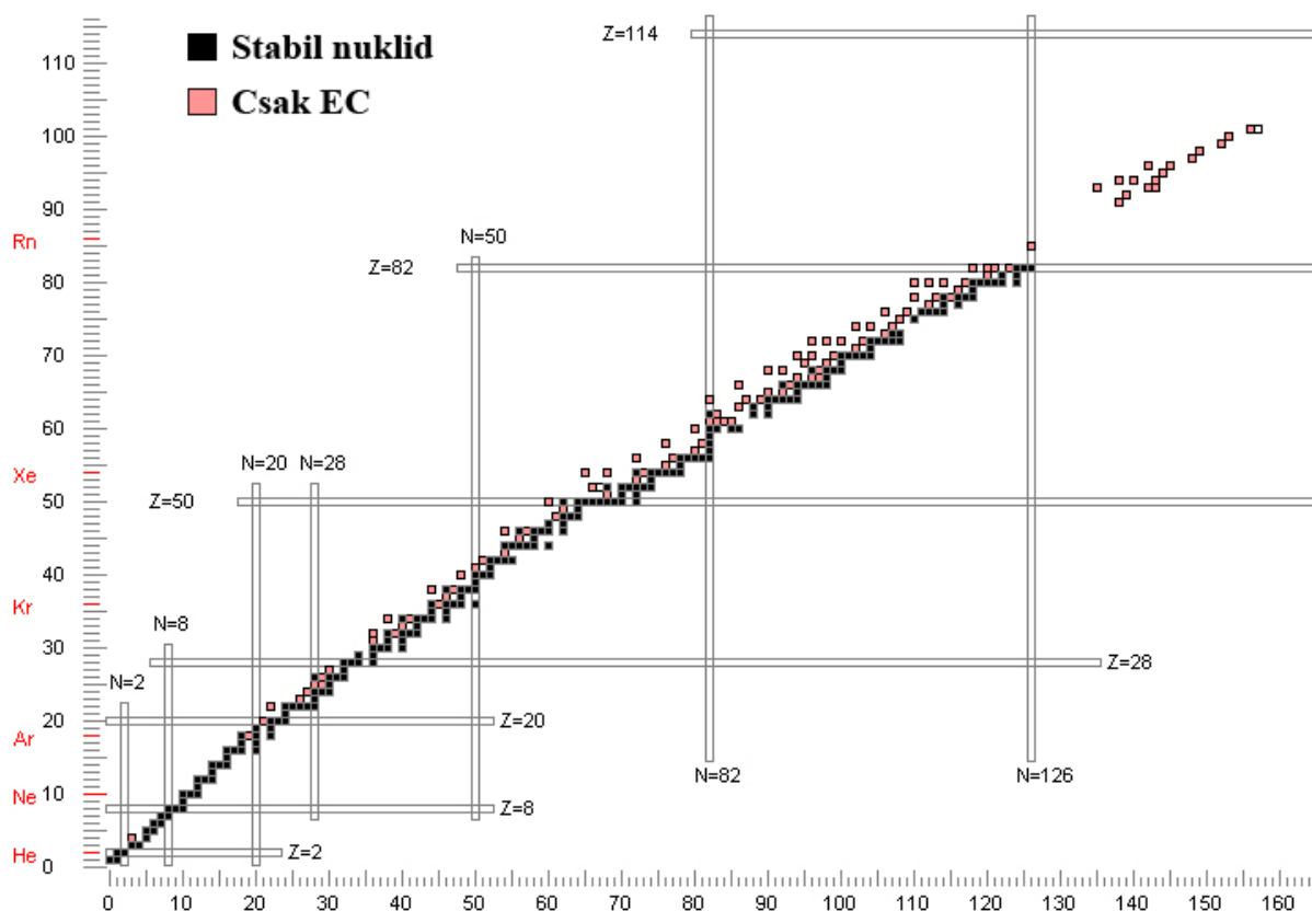
41. ábra: Ez az ábra a Nucleonica ( https://nucleonica.com/ ) Nuclide Explorer funkciójával készült. Csak kétfajta nuklidot választottam ki megjelenítésre, nevezetesen a stabilakat, valamint azokat az instabilakat, amelyek kizárólag EC útján tudnak elbomlani. Nyilvánvaló tendencia érzékelhető az ábrából, ti. az, hogy az EC főleg nehéz magoknál fordul elő, amelyek térfogata sokkal nagyobb átfedésben van a héjelektronok hullámfüggvényével, különösen, ami az 1s-héjat (K-elektronokat) illeti.
