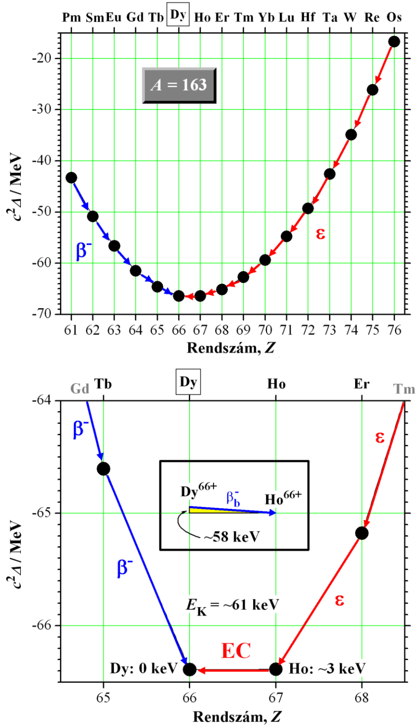
50. ábra: Tipikus páratlan- A tömegparabola a ^{163}\text{Dy} nuklid izobárjaival (felső panel). Az alsó panel a parabola csústartományát nagyítja ki. Az instabil ( T_{1/2} = 4570 \text{ a} ) ^{163}\text{Ho} atom nyugalmi energiája (tömege) mindössze \sim 3 \text{ keV} -vel több a stabil ^{163}\text{Dy} atoménál. (Ez a kis különbség csak az EC-t teszi lehetővé. A \beta^+ -bomláshoz legalább 2 m_e c^2 \approx 1,02 \text{ MeV} tömegcsökkenés szükséges, ami kb. megfelel az alsó panel vízszintes rácsvonalai közt mértnek.) Ez a 3 \text{ keV} jellemzi a magtömegek közti különbséget is. Ugyanakkor a K-héj kötési energiája ( \sim 61 \text{ keV} a hidrogénszerű ^{67}\text{Ho}^{66+} -ban) sokkal nagyobb. Ezért a csupasz ^{163}\text{Dy}^{66+} mag \beta_b -bomlást szenvedhet, mert kb. nettó 61 \text{ keV} - 3 \text{ keV} = \sim 58 \text{ keV} energia szabadulhat fel, miközben a Dy elbomlik, s a keletkező elektron befogódik a keletkező Ho üres K-héjára. A belső ábrán látható, \beta_b -bomlást jelképező kék nyíl lejtése nagyjából arányban van a panelen lévő többi nyíléval.
