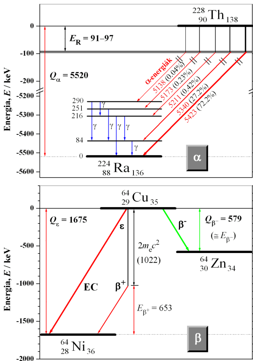
36. ábra: Egyszerűsített bomlási sémák alfa- és béta-bomlásra. A számértékek energiát jelentenek keV egységben. A felső panelen szereplő \alpha -bomló ^{228}\text{Th} 4n+0 természetes bomlási sor (51. ábra) második tagja. A sémán jól látszik az \alpha -bomlás egyik jellegzetessége, nevezetesen, hogy az elágazási arányok (%-értékek) igen erősen függenek az \alpha -energiától: minél nagyobb E_\alpha , annál „erősebb” az illető ág az \alpha -csoporton belül. (Lásd a Geiger–Nuttall-grafikont a 19. ábrán.) A leány szintdiagramja messze nem teljes. (A részletes bomlási sémát gyakorlásképpen keresse meg a nudat3 webhelyén, ahonnan az ábrához felhasznált 2012-es adatokat vettem. Vagy ami még jobb, menjen a Live Chart of Nuclides oldalra, a 12C helyére írja be a ^{228}\text{Th} nuklidkódot, majd nyomja meg a Q ikont és végül a Decay Radiation fület.) Itt csak azok a szintek szerepelnek, amelyek az anyanuklid \alpha -bomlása során keletkeznek. Vegyük észre azt is, hogy a Q -érték \sim 1,8\% -a leányatom E_R visszalökődési energiájaként jelenik meg. (Minél nagyobb E_\alpha , annál nagyobb E_R : ennek köszönhető annak a „szintvonalnak” az elmosódottsága, amelyből a piros ferde nyilak kiindulnak.) Megjegyzendő: ez a kis energiátörredék még így is csaknem 100 keV, melynek hőmérséklet-egyenértéke \sim 1 GK. Ez azt jelenti, hogy a visszalökődött atomok meglehetősen „forrók”. A \beta -bomló ^{64}\text{Cu} is egyike a félszáz páratlan- Z & páratlan- N típusú nuklidnak, amelyek mind \beta^- (39%), mind \epsilon (61%) bomlásra hajlandóak. (Lásd az 58. ábra spektrumait.) Az \epsilon -ág maga is két ágra bomlik ebben az esetben: \beta^+ (17,4%) és EC (43,6%) egyaránt lehetséges, ha nem is egyforma valószínűséggel.
