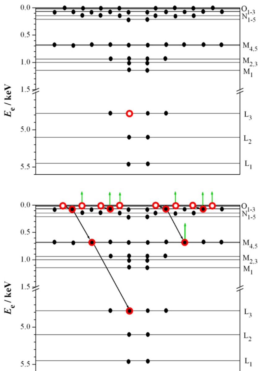
59. ábra: Auger-kaszád kialakulása egy belső lyukkal rendelkező ^{54}\text{Xe}^+ ion példáján szemléltetve. A példában szereplő \text{Xe}^+ egyetlen elektronlyukat tartalmaz az L-héjon (felső panel), majd a lavinaszerű Auger-effektus-sorozat (Auger-kaszád) következtében \text{Xe}^{8+} ionná alakul, melynek O-héja ezáltal teljesen „lecsupaszodik” (alsó panel). A (fekete) ferde nyilak egy-egy belső lyuk betöltését jelzik egy kintebbi elektron által, miközben a lyuk kijebb vándorol. A lyukbetöltés közben felszabaduló energiát egy elszabaduló héjelektron (Auger-elektron) viszi el kinetikus energia formájában (l. a függőleges zöld nyilakat). Az Auger-elektron által visszahagyott lyuk hasonlóan töltődhet be, így a lyukak számát (ideális esetben) a kaszkád minden lépcsője megduplázza. Eközben a keletkezett lyukak héjról héjra kifelé vándorolnak, míg el nem érik a vegyértékhéjat (mely az O-héj ezúttal). A mechanizmusból következik, hogy az Auger-elektronok energiaspektruma, a karakterisztikus röntgensugárzáshoz hasonlóan, jellemző az illető kémiai elemre, minthogy mindkettőt az érintett elektronok kötési energiái ( E_e ) határozzák meg.
