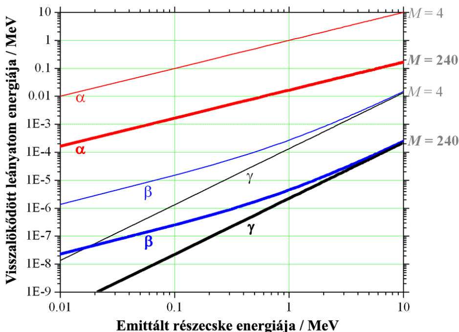
56. ábra: A leányatom visszalökődési energiája a sugár részecske ( \alpha , \beta , ill. \gamma ) kinetikus energiája függvényében egyrészecskés emisszió esetében. A görbéket két extrém esetre számítottam, nevezetesen egy nagyon könnyű leányatomra M = 4 nuklidtömeggel (vékony vonalak) és egy nehézre M = 240 nuklidtömeggel (vastag vonalak).
