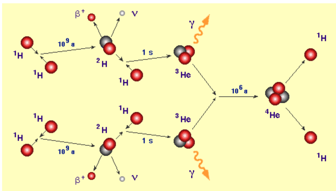
79. ábra: A pp I lánc a hidrogénégés tipikus mechanizmusa a Napéhoz hasonló tulajdonságú fősorozatbéli csillagokban . A sebességmeghatározó lépés az első reakció, mely deutérium ( {}^2\text{H} ) képződéséhez vezet. A pp II és pp III folyamat a Nap maghőmérsékletéhez képest egyre forróbb körülmények között jut csak szerephez. (Rick Firestone ábrája alapján)
